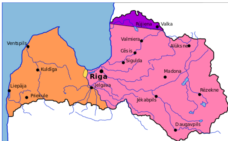
16. april 1919: I march foretog de forenede tyske og lettiske styrker (orange og gul) et modangreb og erobrede det meste af kysten
