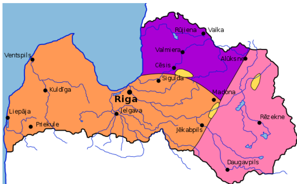
22. juni 1919: Den 3. estiske division (purpur) angriber de tyske tropper ved Cēsis i starten af juni og vinder slaget den 23. juni
